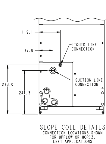
Fig. 3 – PF4MNB – Metric
