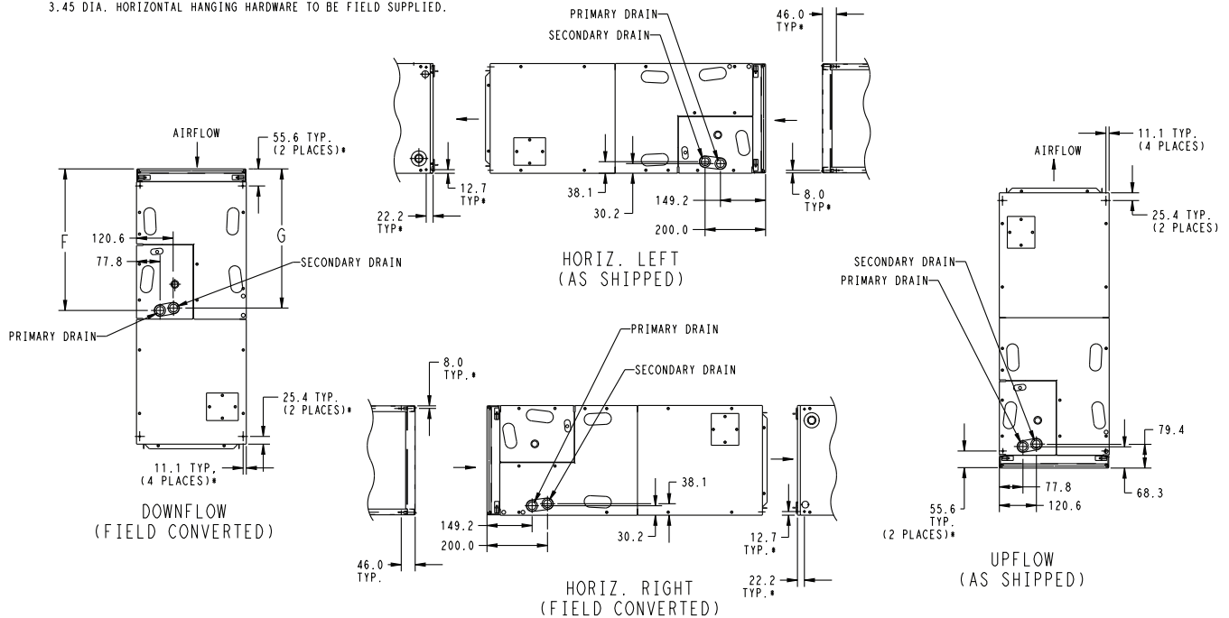
Fig. 4 – PF4MNB – Metric
